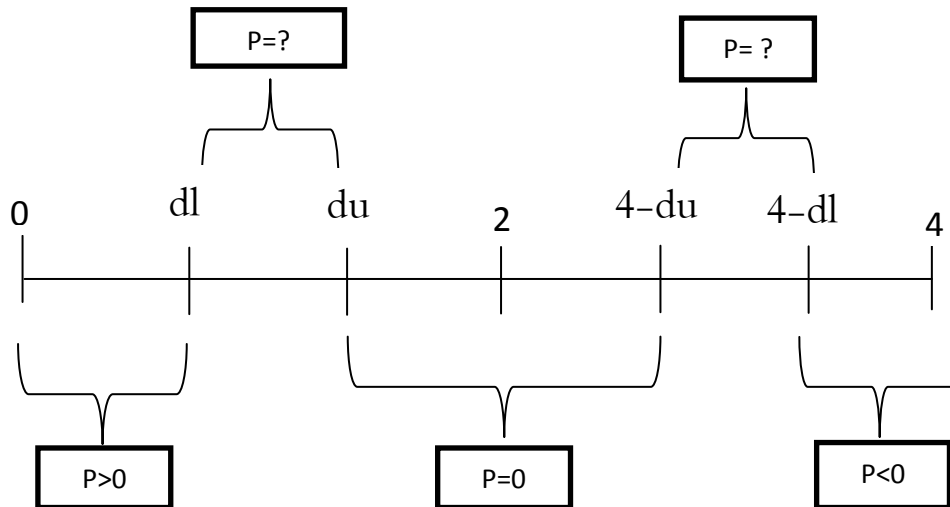
الشكل (18) : مناطق القبول والرفض لاختبار "Durbin- watson"
