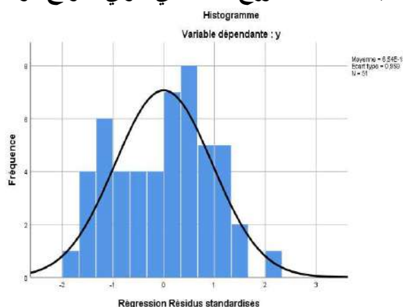
الشكل (15): اعتدالية التوزيع الاحتمالي لبواقي نموذج مؤسسة Condor
