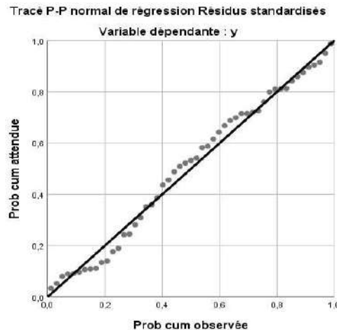
الشكل(16):الانتشار الخطي لبواقي نموذج مؤسسة Condor
